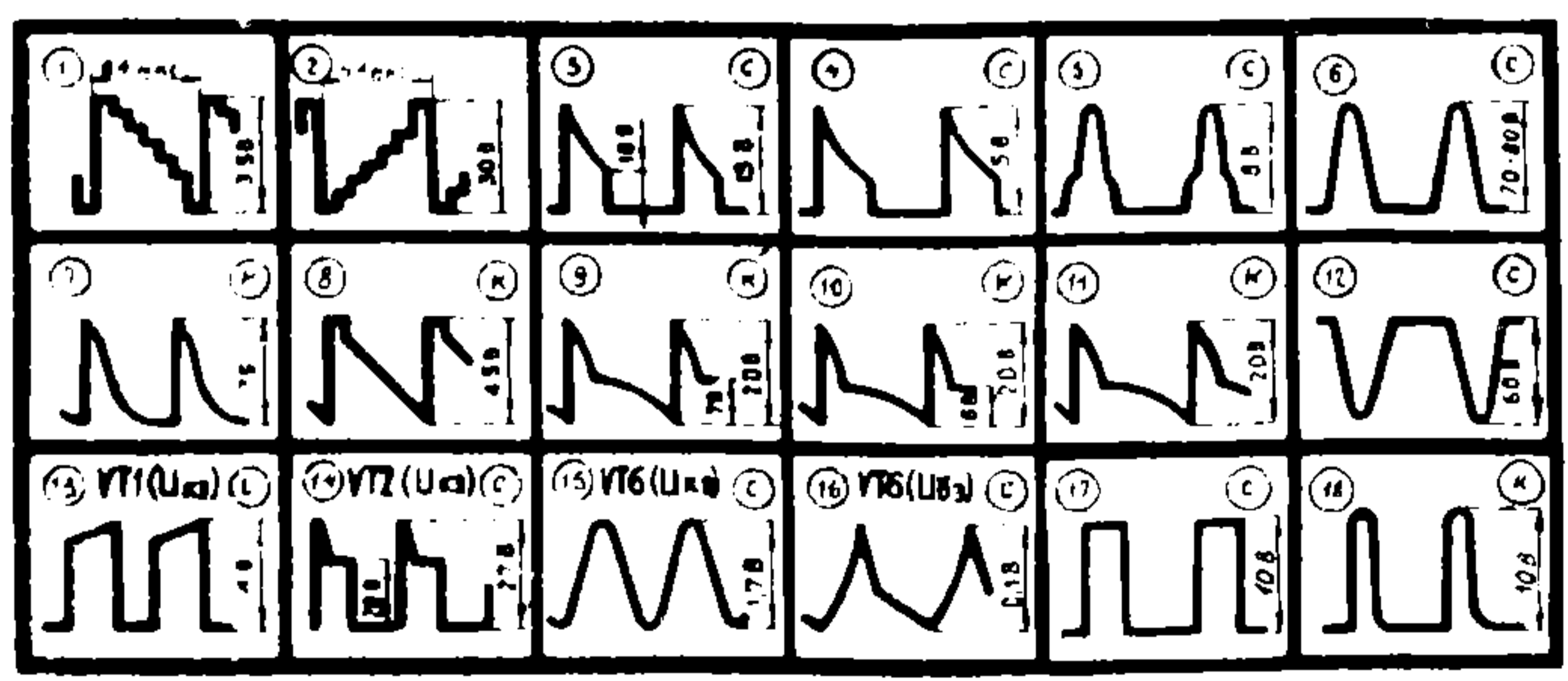
ОСЦИЛЛОГРАММЫ НАПЯЖЕНИЙ
